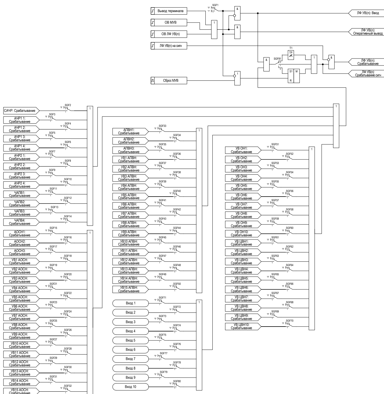
Рисунок 2.21 – Функциональная схема МУВ
